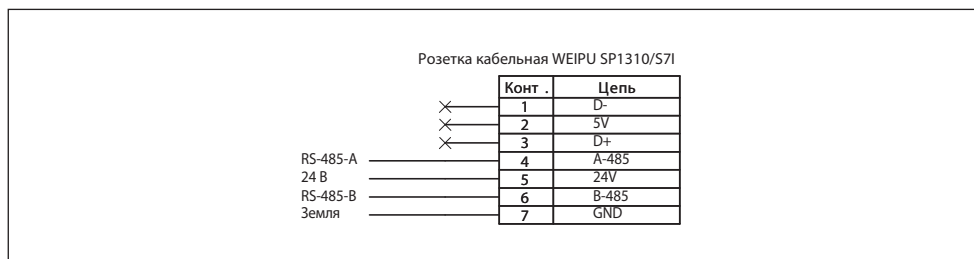
Рис.3. Схема распылки коннектора при подключении к сети электропитания 24 В и сети передачи данных на основе RS-485.
