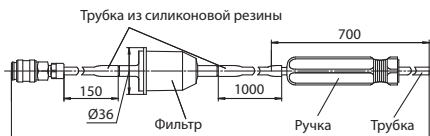
Рис.4. Пробоотборные устройства
