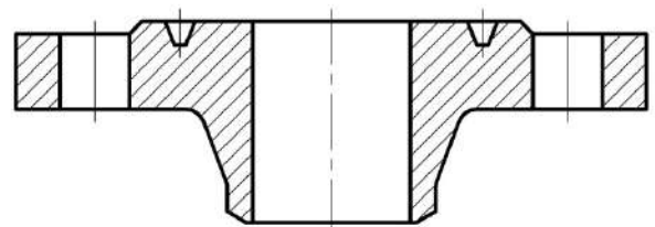
J – под прокладку овального сечения
