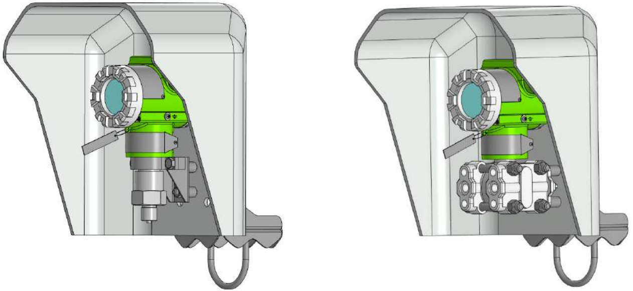
Рисунок И.6 – Внешний вид защитного козырька для датчика давления ЭМИС-БАР с использованием углового кронштейна
