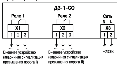
Рисунок 3 – Функциональное назначение клемм прибора
