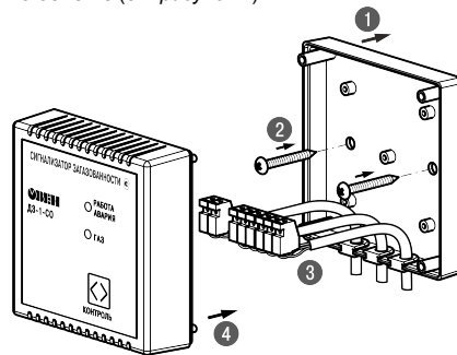
Рисунок 2 – Монтаж прибора
