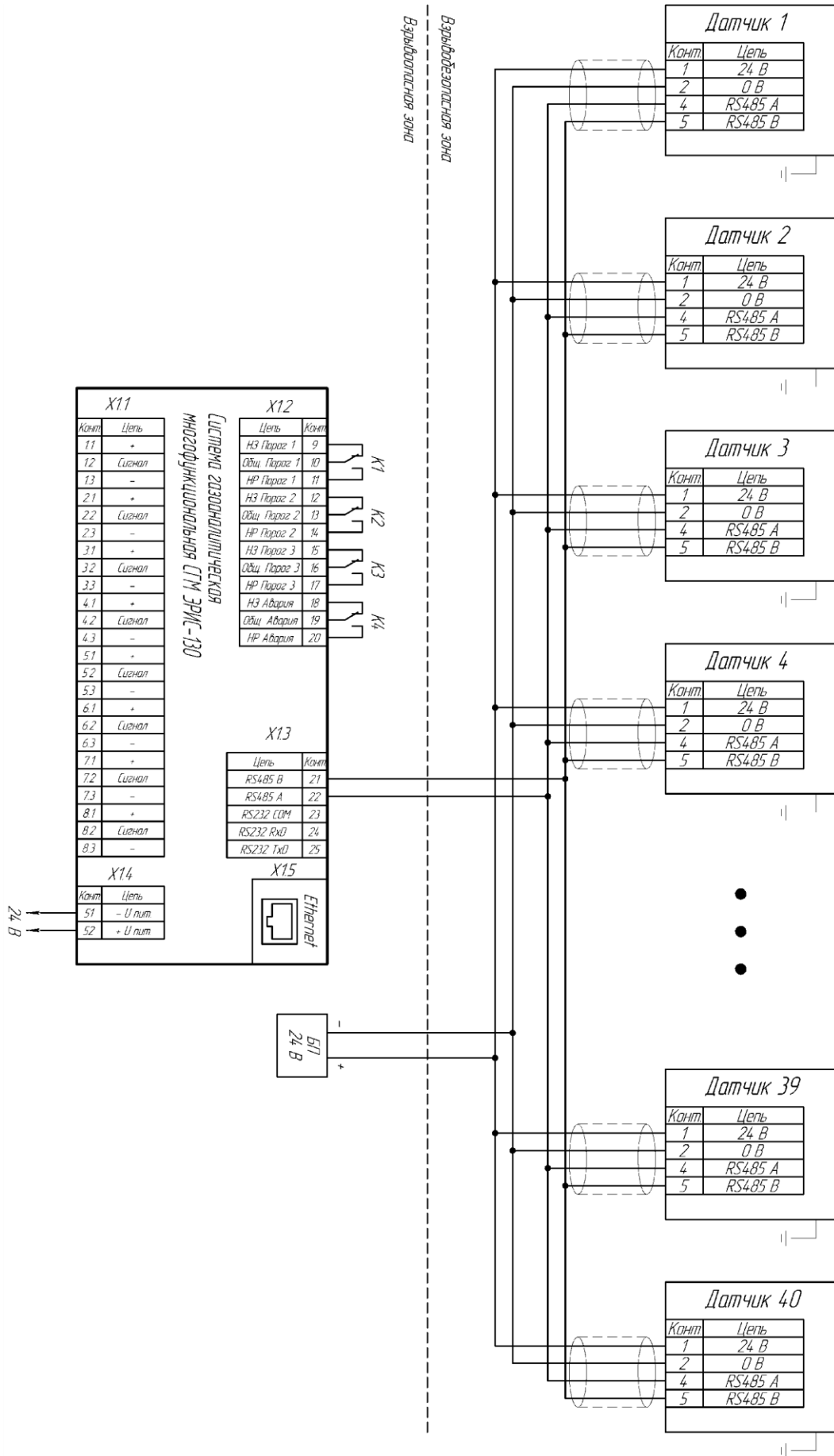
Рисунок Б.2 - Принципиальная схема подключения ЭРИС-130. Подключение датчиков по интерфейсу RS485 Modbus RTU
