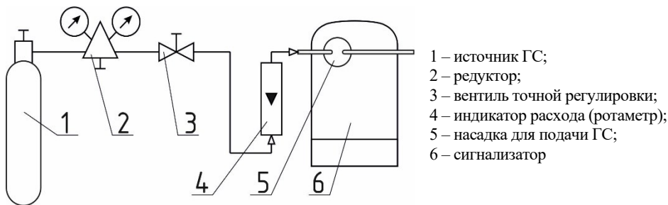
Рисунок Г.1 – Схема подачи ПГС
