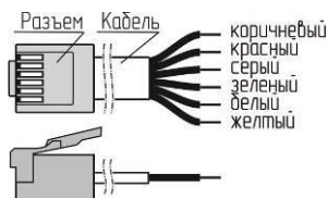
Вилка на кабель TP6P6C
